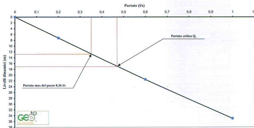
Fig. 7 - Grafico LP \rightarrow Q relativo ad un acquifero tipicamente artesiano con esistenza di una portata critica.
