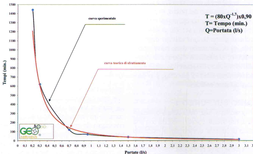
Fig. 5 - Curve sperimentali e teoriche (curve T \rightarrow Q ) di sfruttamento del pozzo.
