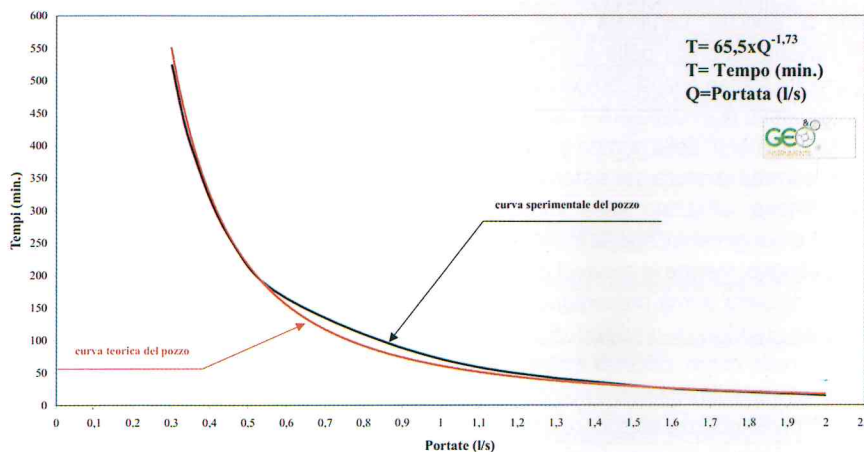
Fig. 6 - Curve sperimentali e teoriche (curve T \rightarrow Q ) di sfruttamento del pozzo.
