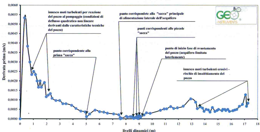
Fig. 4 - Pozzo "Sulfureo 1" - abbassamenti piezometrici in funzione del tempo di pompaggio (LP → t) relativi alla prova di lunga durata; la curva mostra chiaramente la posizione delle sacche di alimentazione laterale dell'acquifero e il punto di inizio del collasso del pozzo.
